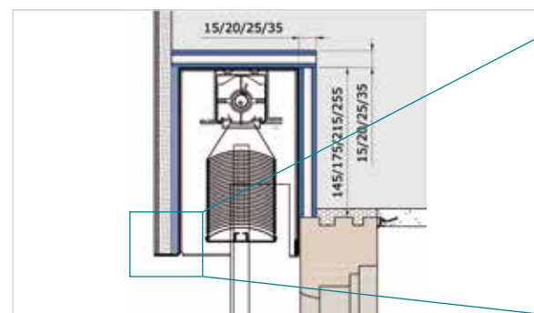
Mit Sturzaussparung und Sturzdämmung RAFF S PUTZ
