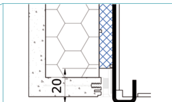
Sonderausführung für Wärmedämmverbundsystem mit Platz zum Anbringen von Anputzleisten
