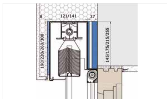
Mit Wärmedämmverbundsystem und Sturzdämmung RAFF S WDVS mit integriertem Rollo
