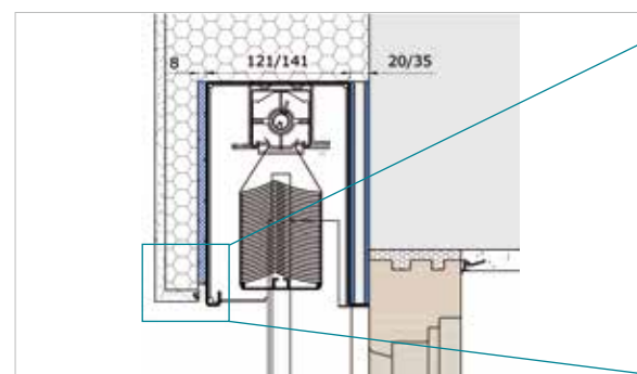
Mit Wärmedämmverbundsystem und Sturzdämmung RAFF S WDVS
