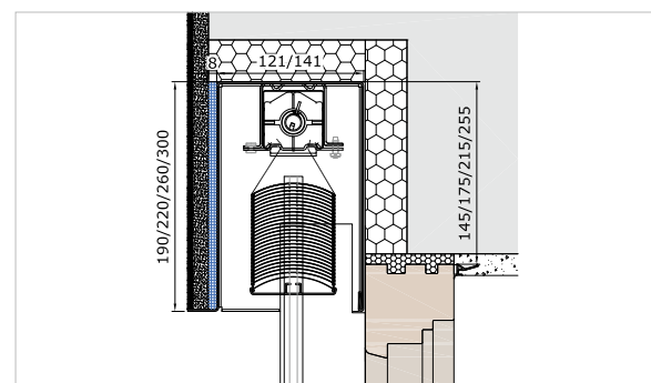
Mit Stockaufdopplung RAFF S PUTZ
